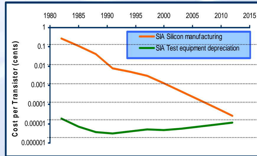
Transistor 당 검사 비용 추이
